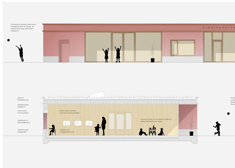
Ansicht, Schnitt
